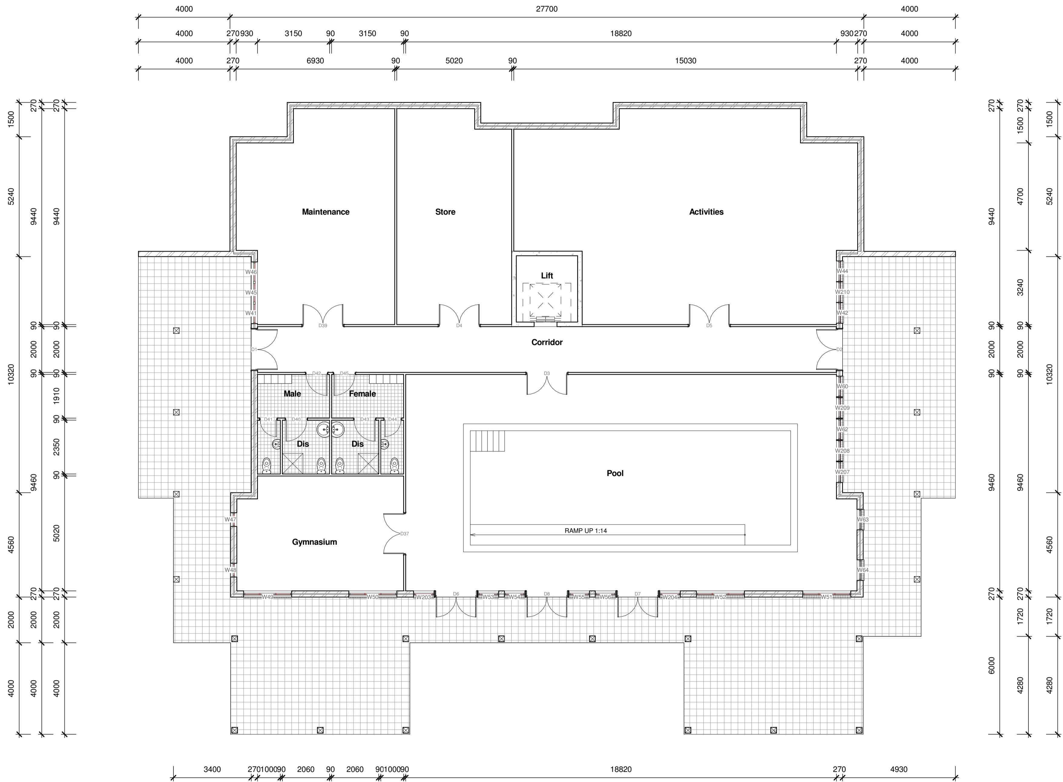
1 Level 1 1 : 100
